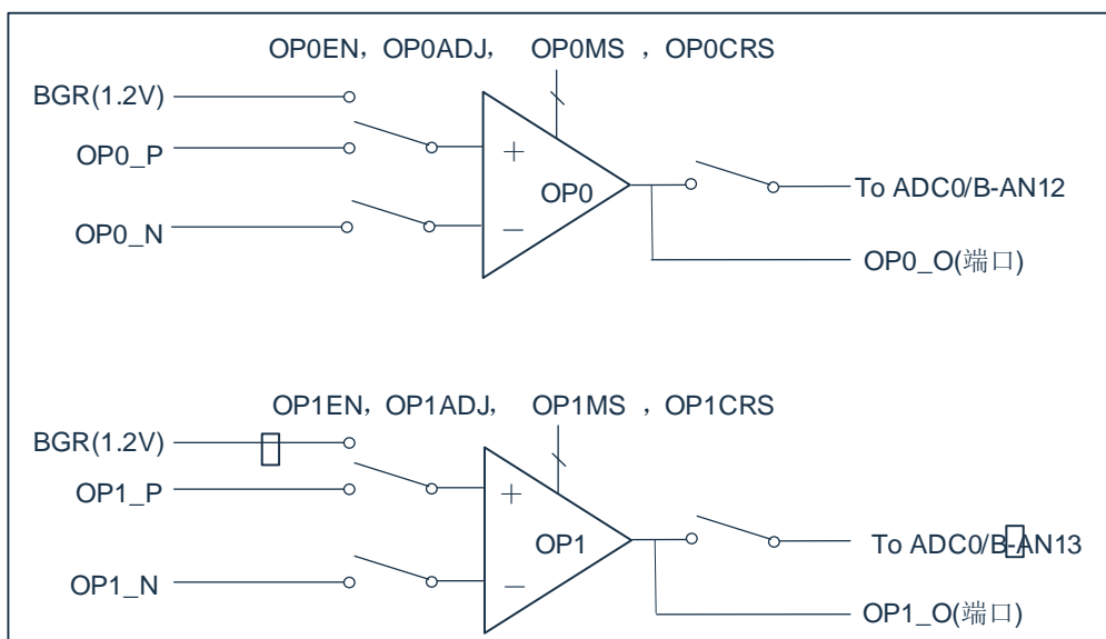
图 22-1: 运放与 PGA 结构图 (1)
