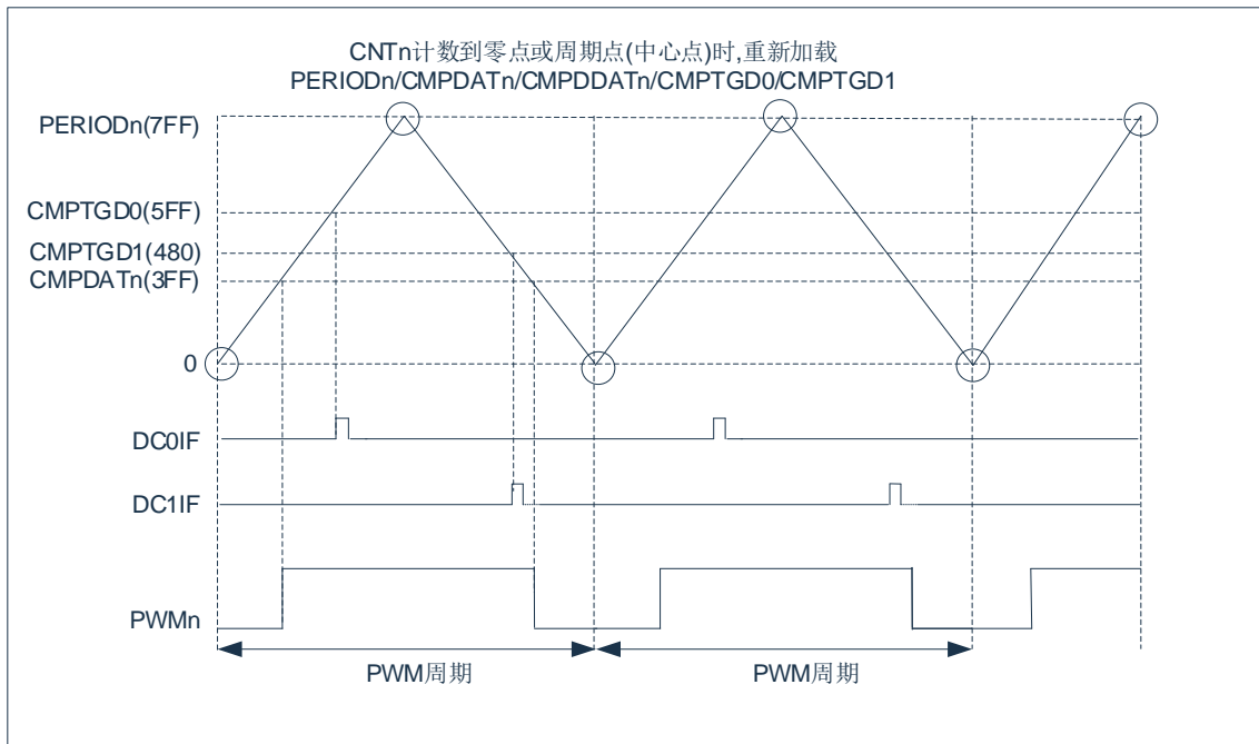
图 16-9: 中心对齐模式，数字比较器的工作方式
