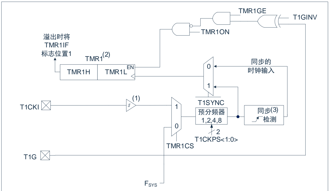
图9-1: TIMER1结构图
