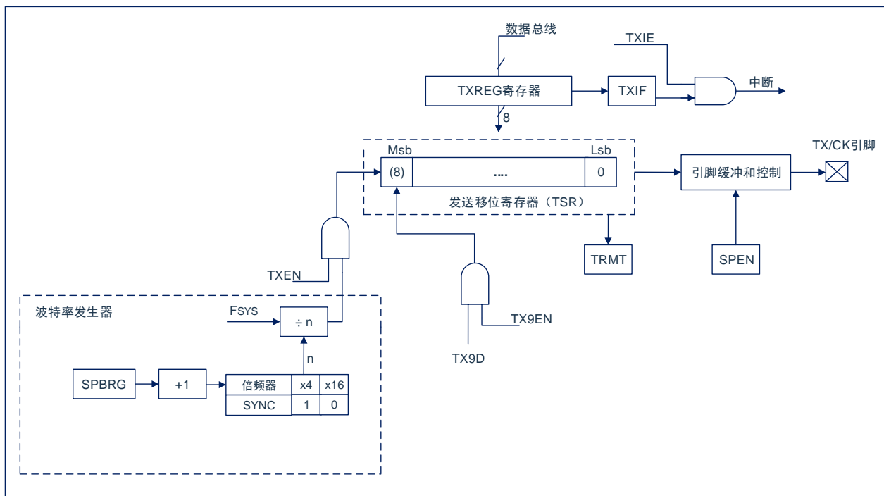
图13-1：USART发送框图
