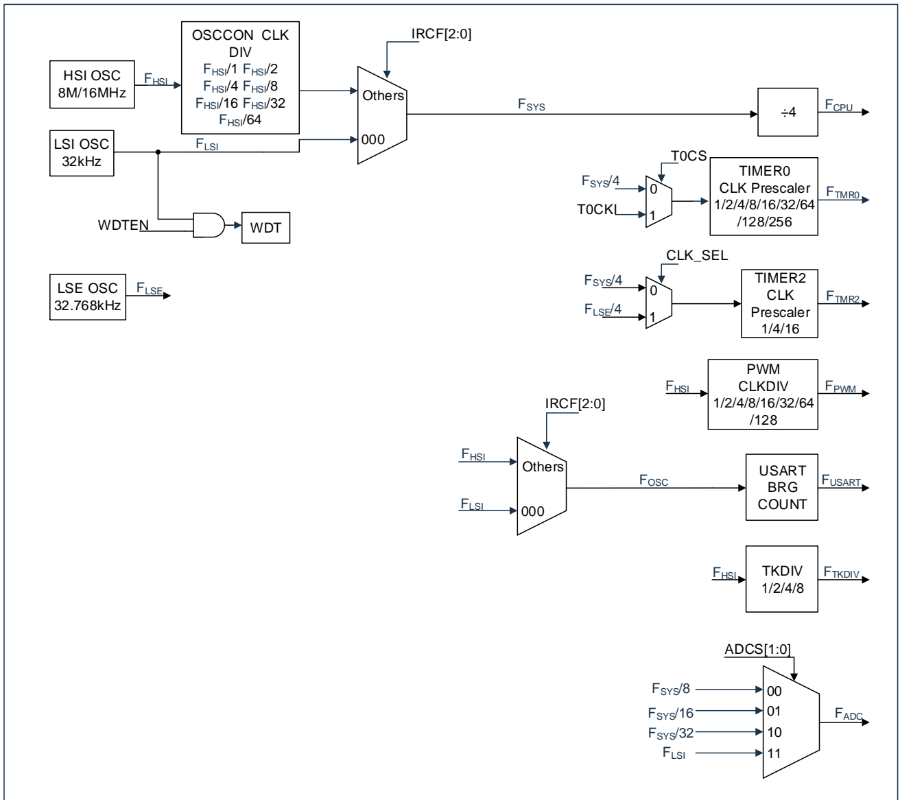
图 3-2: 时钟框图
