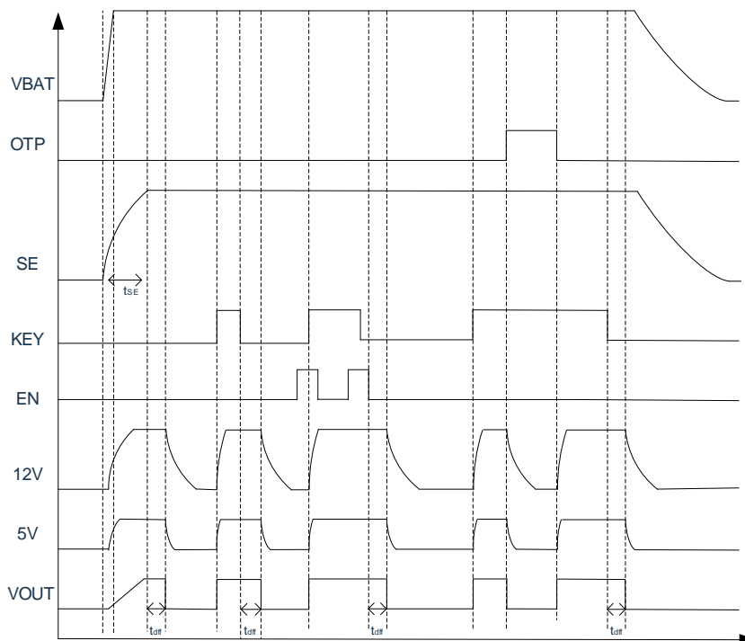
逻辑时序图
