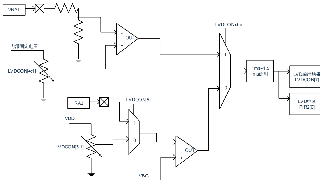
图 15.1: LVD 框图
